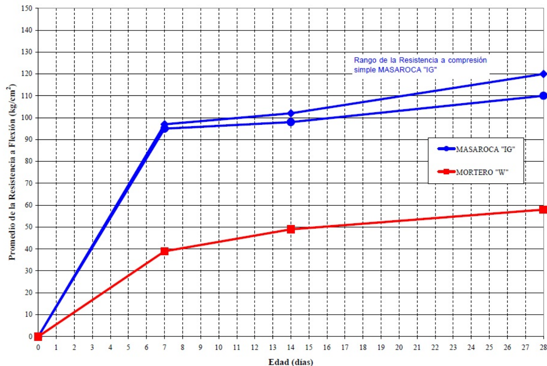
DESARROLLO DE LA RESISTENCIA A FLEXIÓN (VIGAS DE 4cm x 4cm x 16cm)
