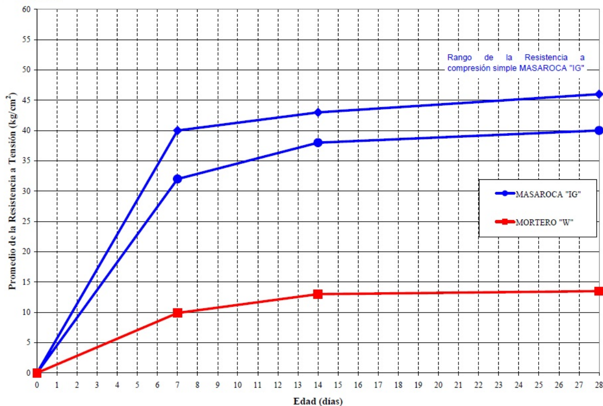
DESARROLLO DE LA RESISTENCIA A TENSIÓN (BRIQUETAS DE 6,5cm 2 SECCIÓN TRANSVERSAL)
